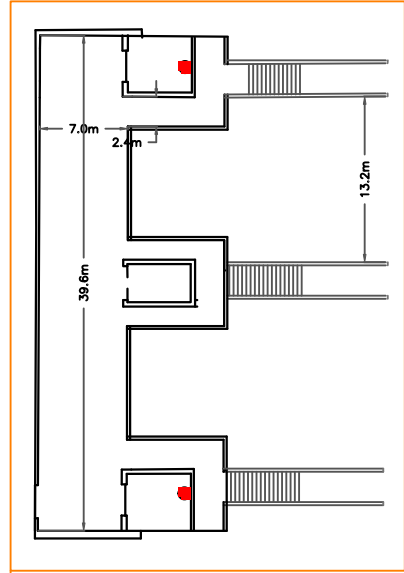
étage mezzanine
